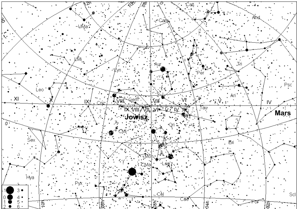
Trasy Marsa i Jowisza na tle gwiazd w 2013 roku.
