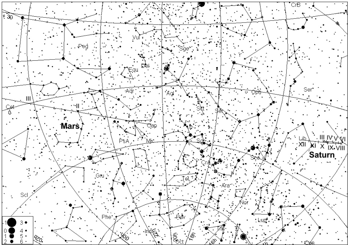
Trasy Marsa i Saturna na tle gwiazd w 2013 roku.
